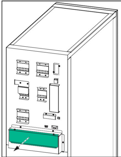
Рисунок 15-13. ИБП мощностью 20 кВА, вид сзади
