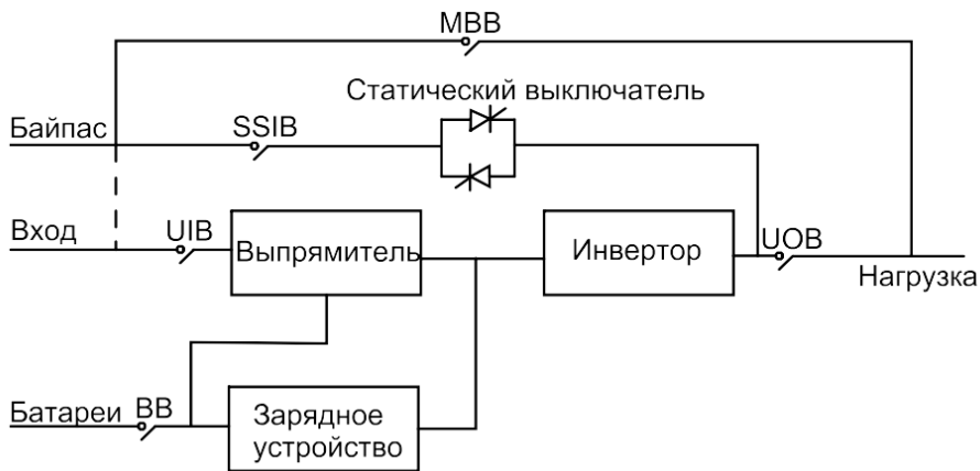
Рисунок 6-1.Одиночный ИБП
