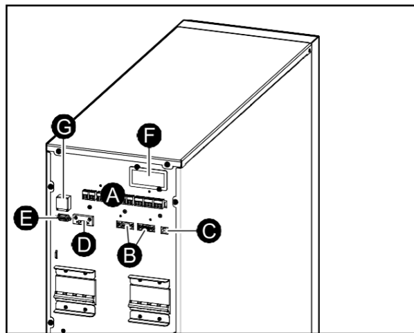
Рисунок 16-2. ИБП 10-15 кВА, 400 В
