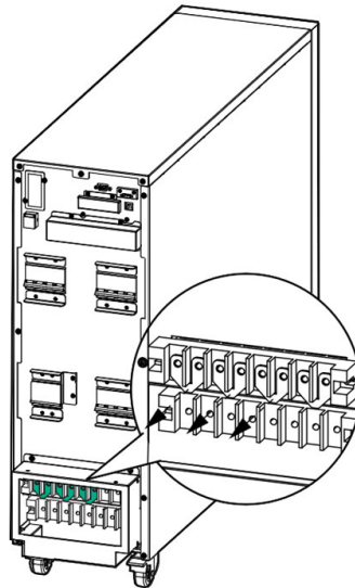
Рисунок 14-8. Одиночный / Двойной ввод
