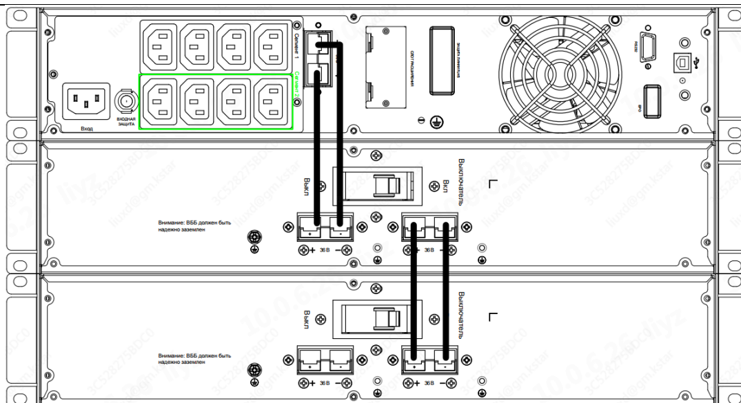
Рисунок 9-10. Установка дополнительных батарейный модулей
