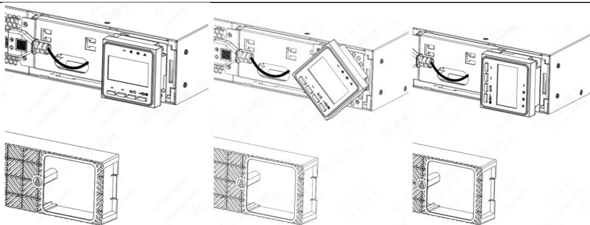
Рисунок 9-6. Установка экрана
