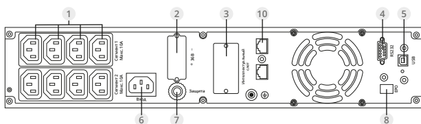
Вид сзади: ИБП ИМПУЛЬС ФРИСТАЙЛ 1500 ВА
