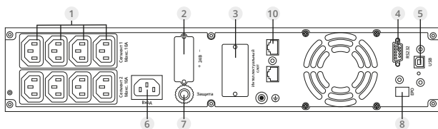
Вид сзади: ИБП ИМПУЛЬС ФРИСТАЙЛ 1000 ВА
