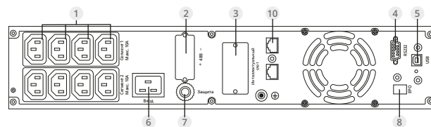
Вид сзади: ИБП ИМПУЛЬС ФРИСТАЙЛ 2000 ВА
